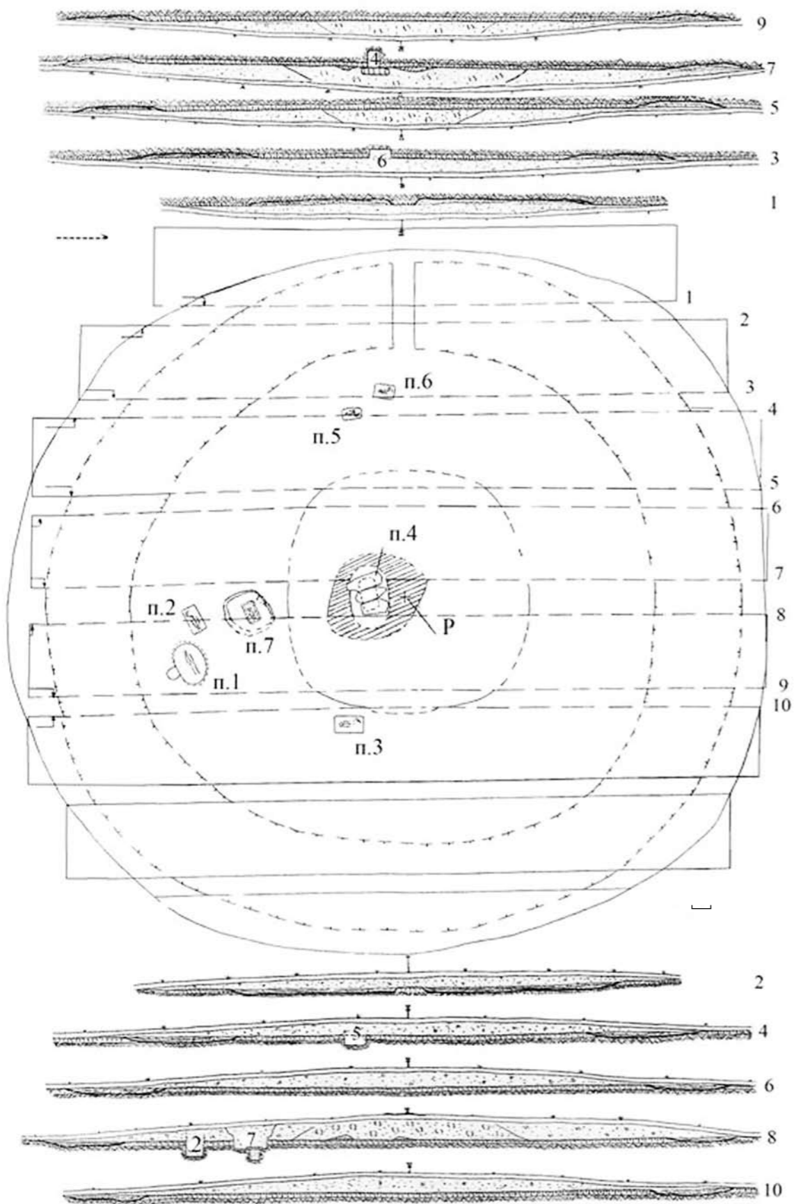
Рис. 2. Общий план кургана у с. Чернобаевка
