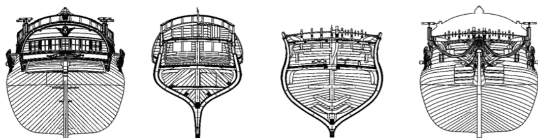
Креслення габари «Le Gros Ventre» 1766 – 1779 рр. в різних проекціях
